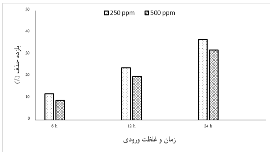
شکل ۳. کارایی تخریب کلروفرم به عنوان تابعی از زمان و غلظت ورودی
