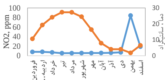
نمودار ۴: الگوی ماهانه آلاینده \text{NO}_2 و دما در ایستگاه پایش آلودگی محیط زیست و ایستگاه هواشناسی بجنورد
