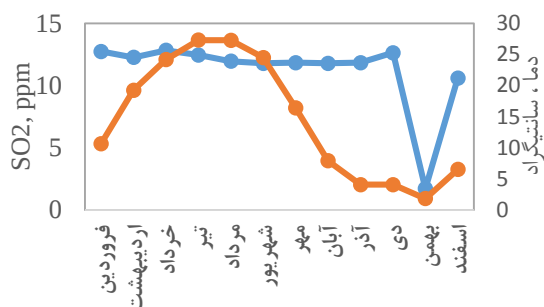
نمودار ۳: الگوی ماهانه آلاینده \text{SO}_2 و دما در ایستگاه پایش آلودگی محیط زیست و ایستگاه هواشناسی بجنورد
